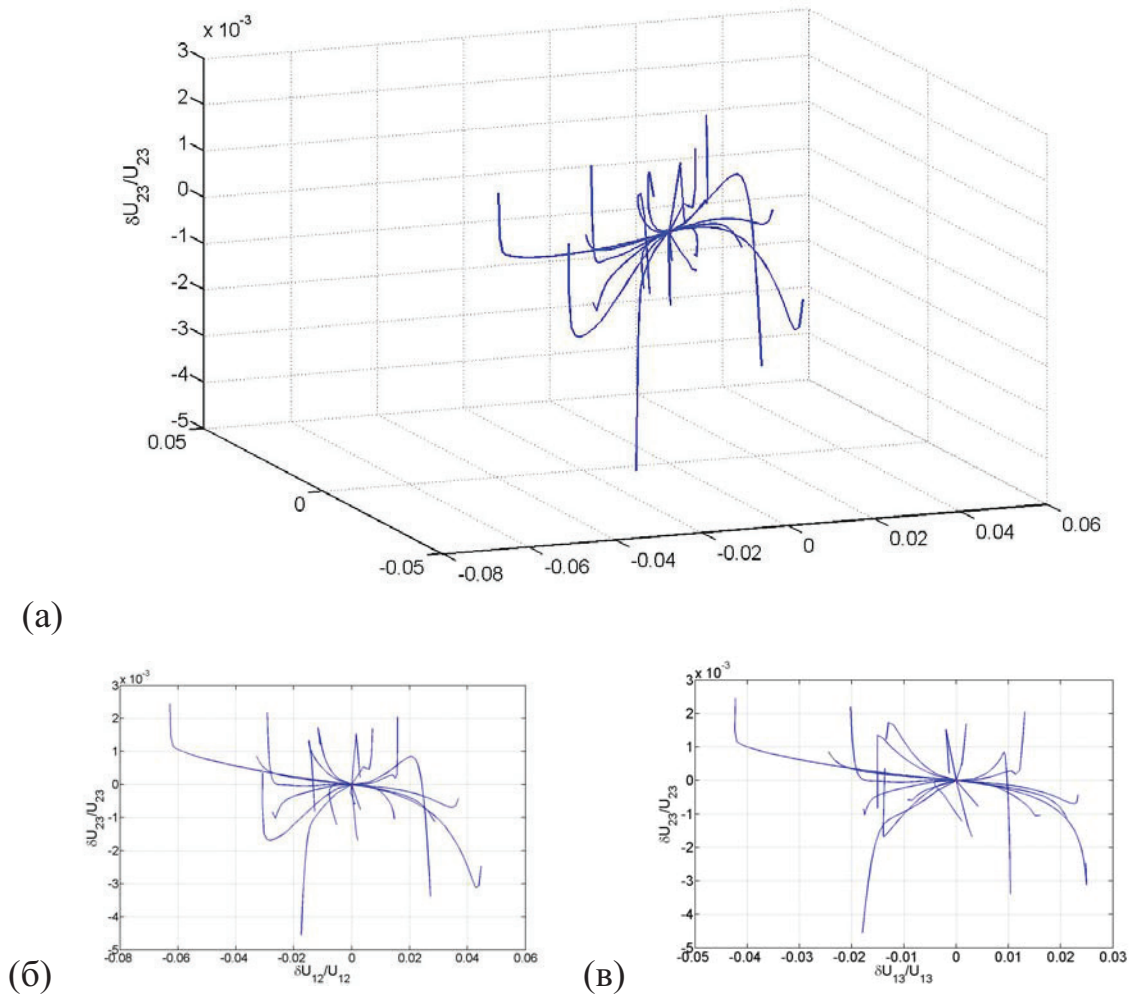
Рис. 20. Динамические траектории образца, представленного на рис. 18а 3D представление, полученное аналогично рис. 3б проекция на оси \delta u_{12}/u_{12}^{(0)} - \delta u_{23}/u_{23}^{(0)} , (в) проекция на оси \delta u_{13}/u_{13}^{(0)} - \delta u_{23}/u_{23}^{(0)} и г) проекция на оси \delta u_{12}/u_{12}^{(0)} - \delta u_{13}/u_{13}^{(0)} .
