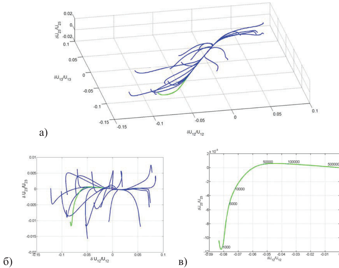
Рис. 35. Динамические траектории, полученные при возбуждении только звеньев активного центра.
